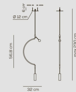
SP LIA P 1 (RECESSED)* kg 1,5 m 3 0,05
