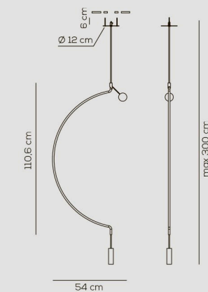
SP LIA G 1 (RECESSED)* kg 2,2 m 3 0,16
